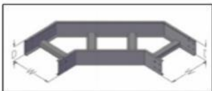
HORIZONTAL ELBOW MULTI-BEND TYPE 1
